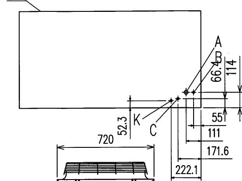
後面 冷媒配管接続口の寸法（平面図）
