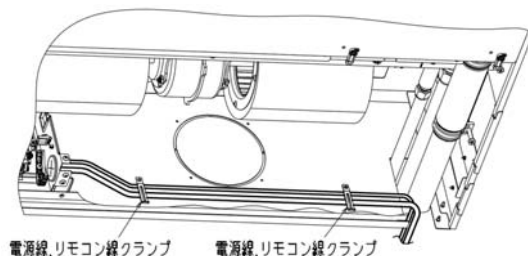
マルチ機の配線接続
