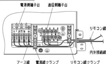
シングル機の配線接続
