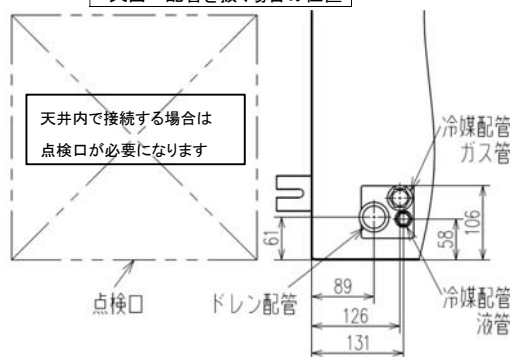
天面へ配管を抜く場合の位置
