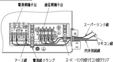
マルチ機の配線接続
