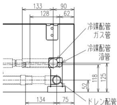
右側面へ配管を抜く場合の位置
