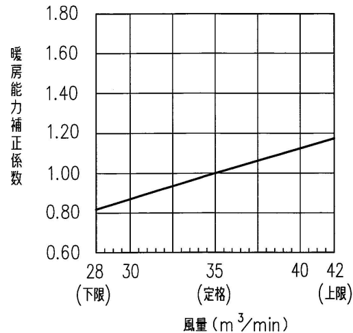
暖房能力特性表
