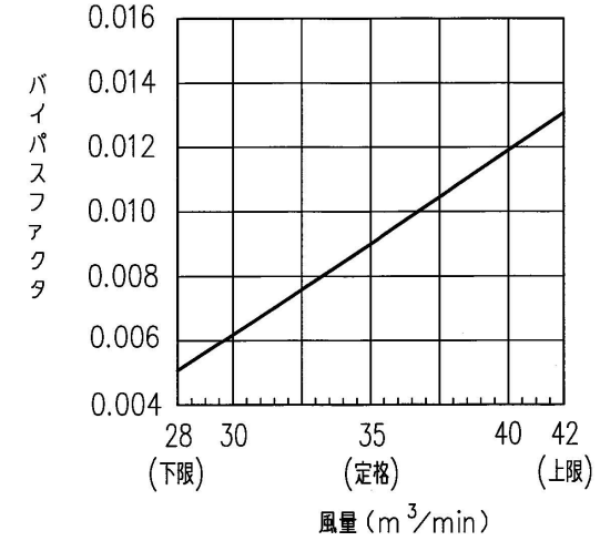
バイパスファクタ表
