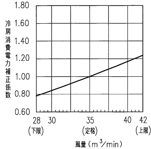
冷房消費電力特性表
