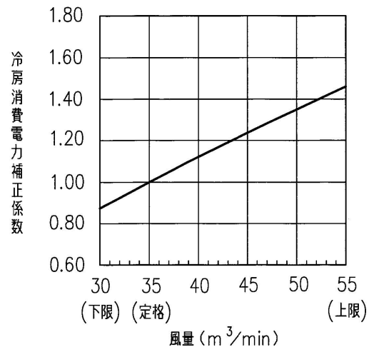
冷房消費電力特性表
