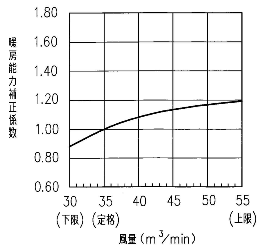
暖房能力特性表
