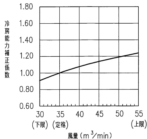
冷房能力特性表
