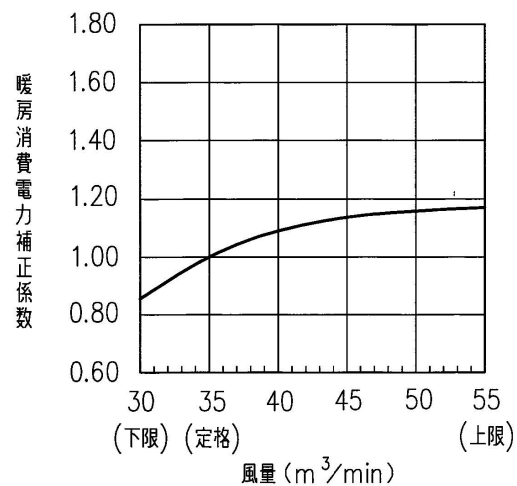
暖房消費電力特性表
