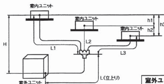
<トリプル機>図A
