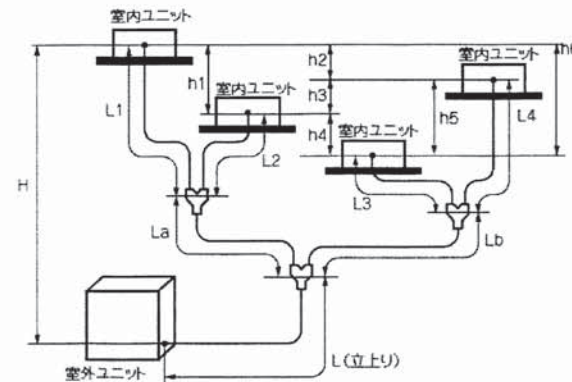
＜Wツイン機＞
