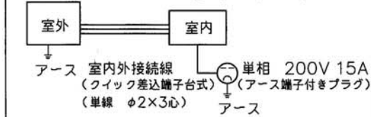
配線接続図
