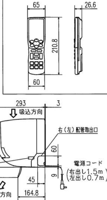
外形図（リモコン）
