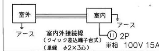
配線接続図
