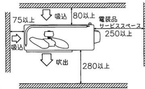
据付スペース（室外ユニット）
