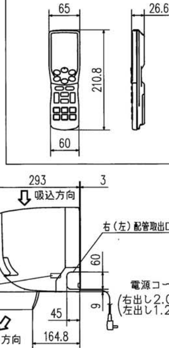
外形図（リモコン）
