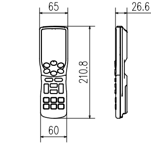
外形図（リモコン）
