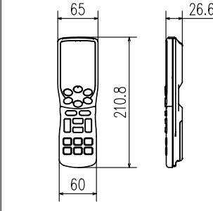
外形図（リモコン）
