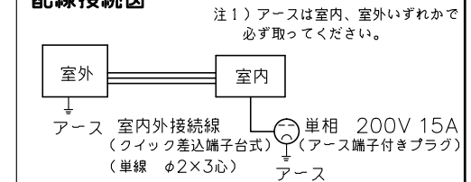
配線接続図
