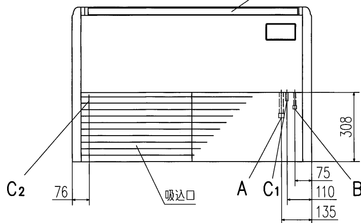
据付スペース
