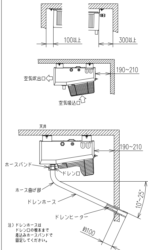
サービススペース (単位: mm)
