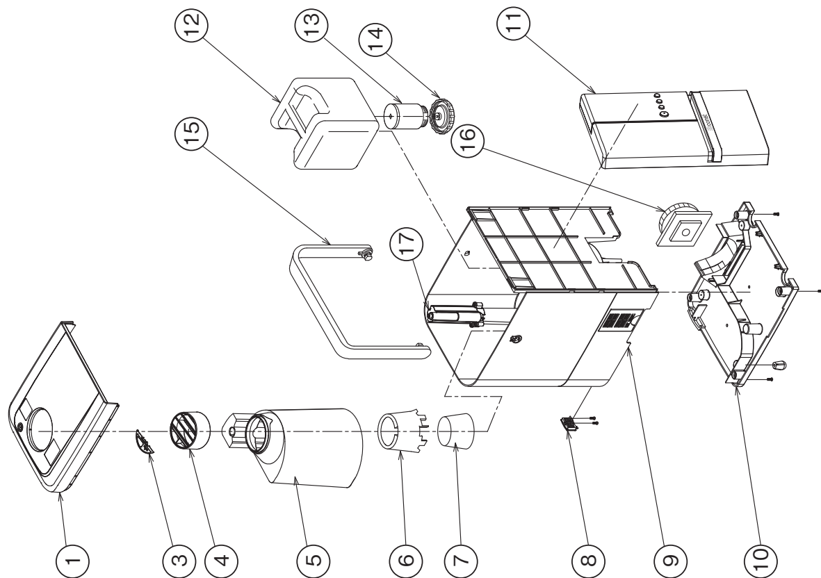
内部詳細図
