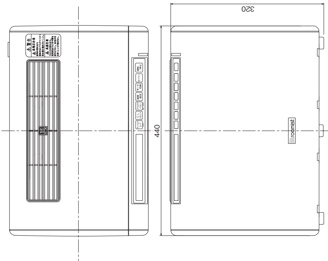
外形図
