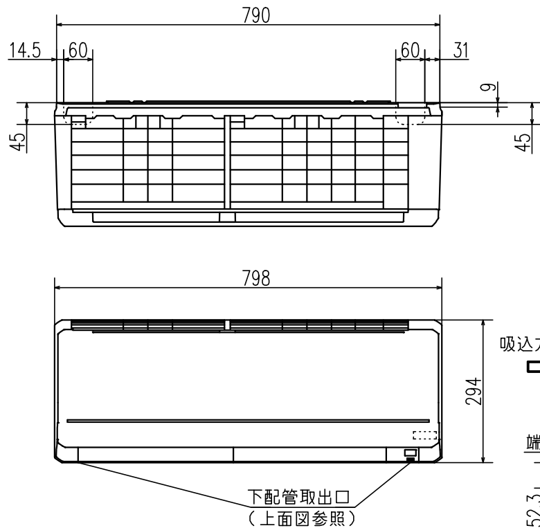
外形図（室内ユニット）
