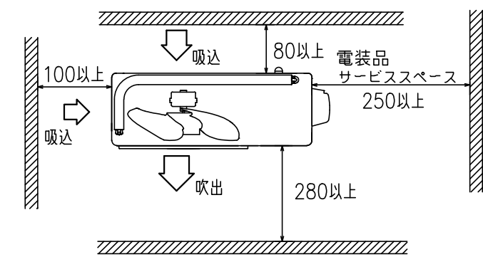
据付スペース（室外ユニット）
