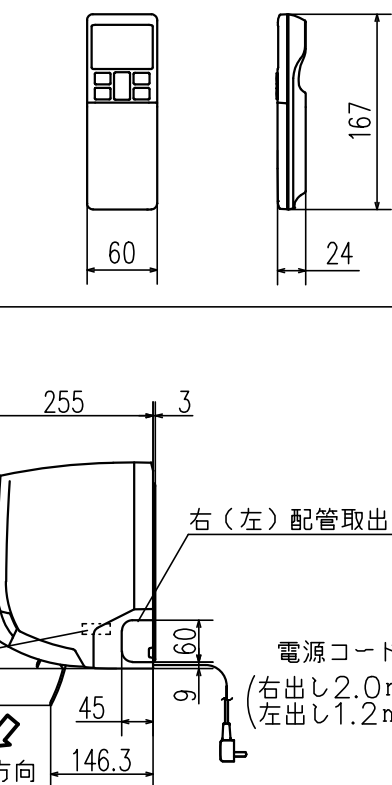
外形図（リモコン）
