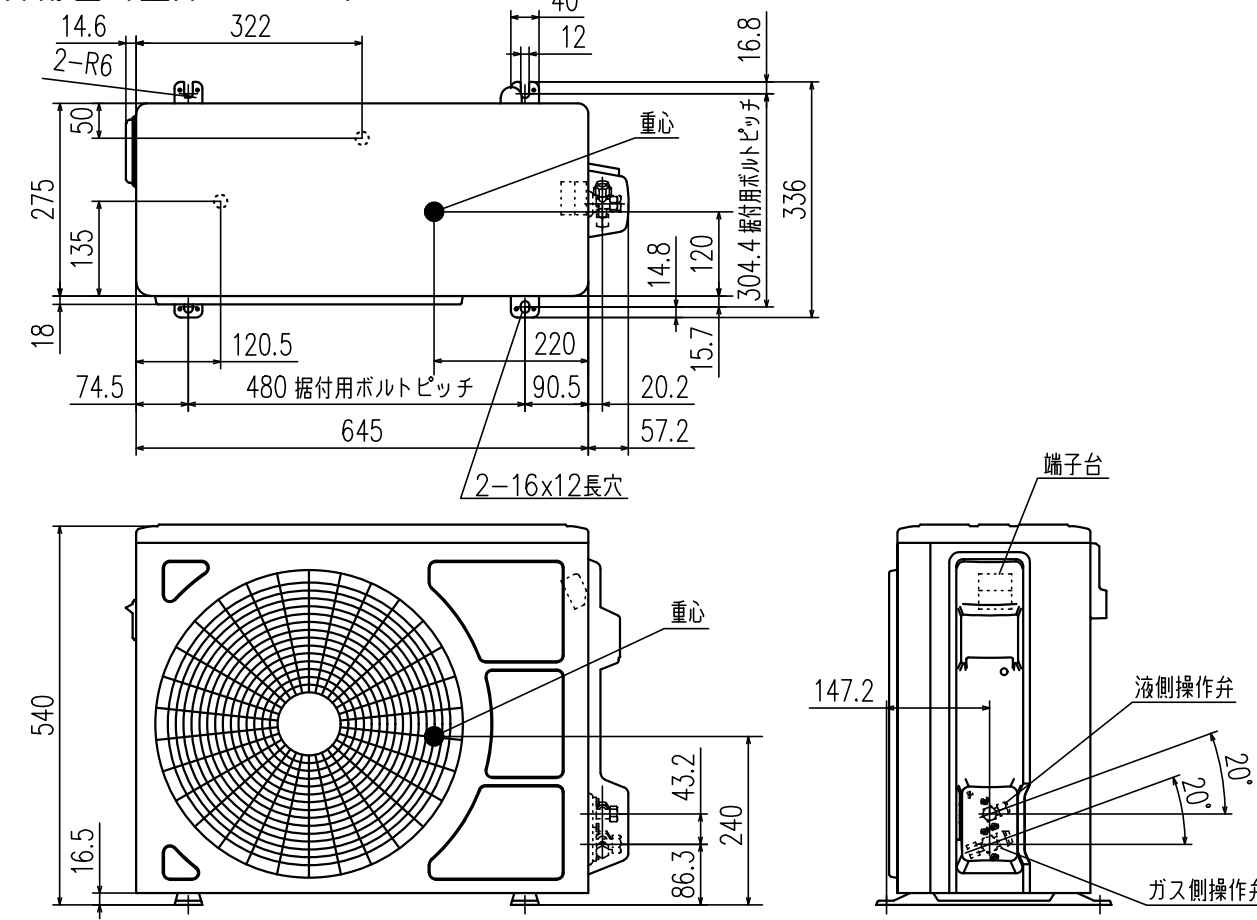
外形図（室外ユニット）
