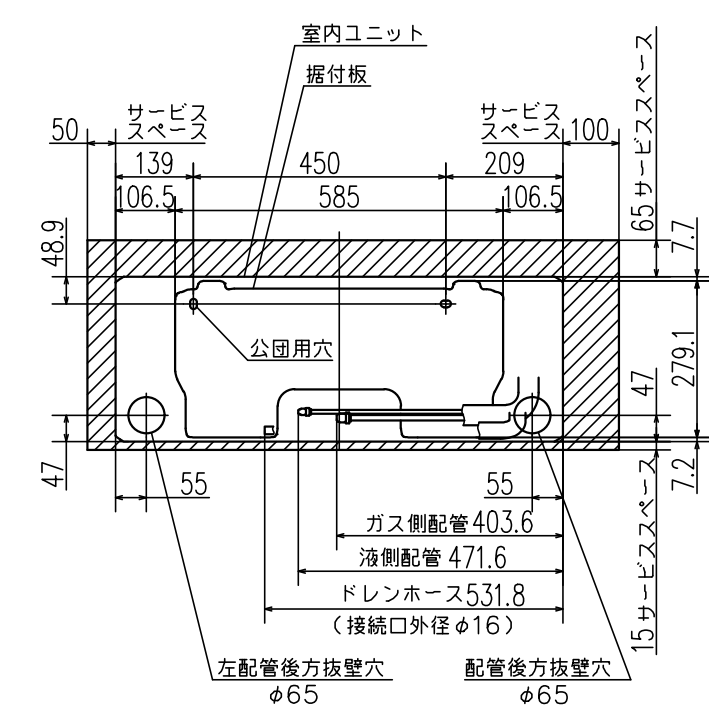
据付スペース（室内ユニット）正面図
