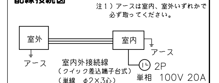
配線接続図
