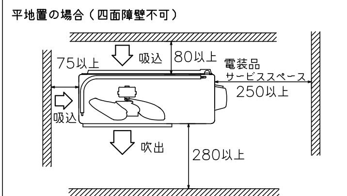
据付スペース（室外ユニット）
