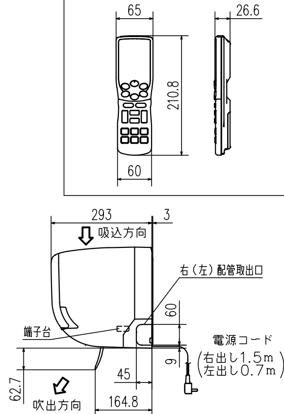
外形図（リモコン）
