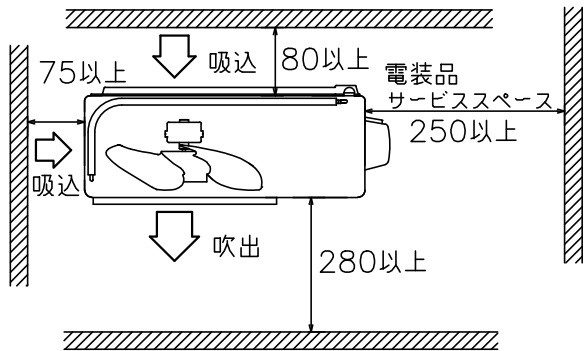
据付スペース（室外ユニット）
