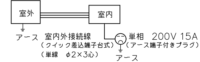
配線接続図
