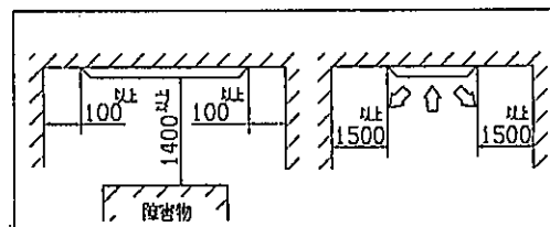
据付スペース
