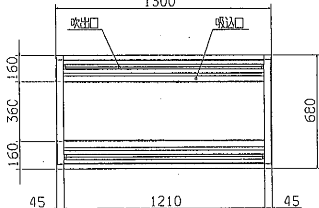
パネル 1300
