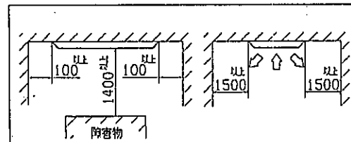
据付スペース
