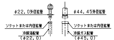
配管接続部詳細
