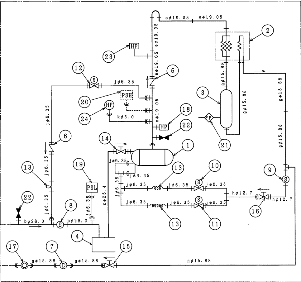
冷凍機
