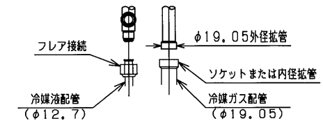
配管接続部詳細
