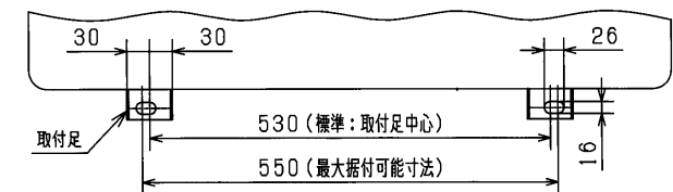
※アンカーボルト用穴詳細
