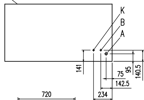
後面 冷媒配管接続口の寸法（平面図）
