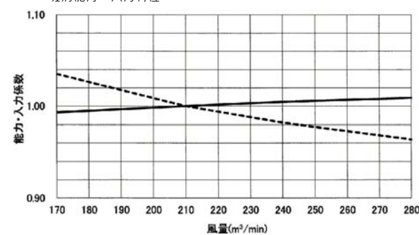
暖房能力・入力特性
