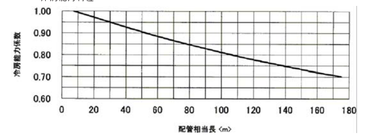
冷房能力特性
