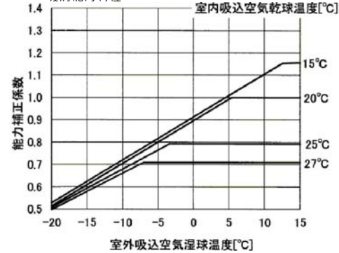
暖房時の室外熱交換器への着霜による補正係数（暖房のみ）
