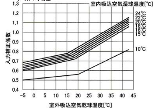
暖房入力補正
