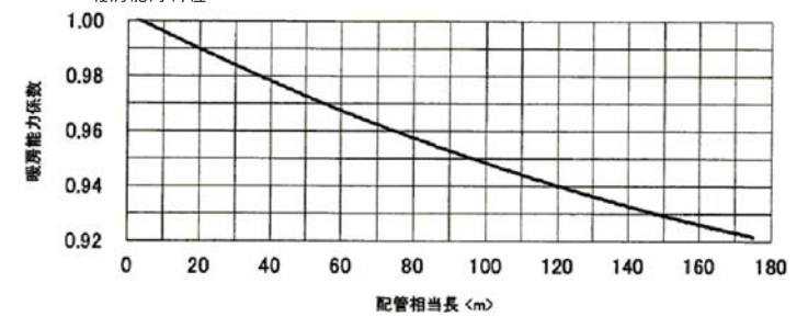
暖房能力特性
