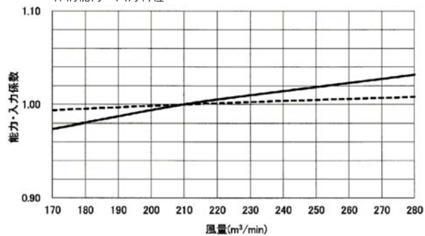
冷房能力・入力特性
