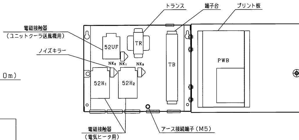
機器配置図
