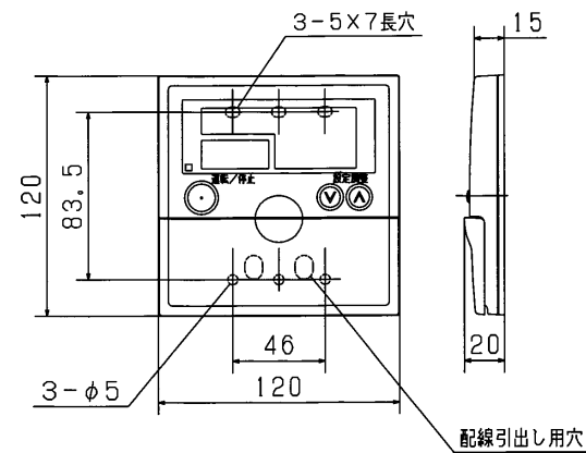
リモコン寸法図
