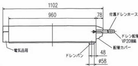
化粧パネル外形図 (TTPN-VX,CX,MX,TX)
