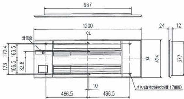
化粧パネル外形図 (TTPN-VX,CX,MX,TX)
