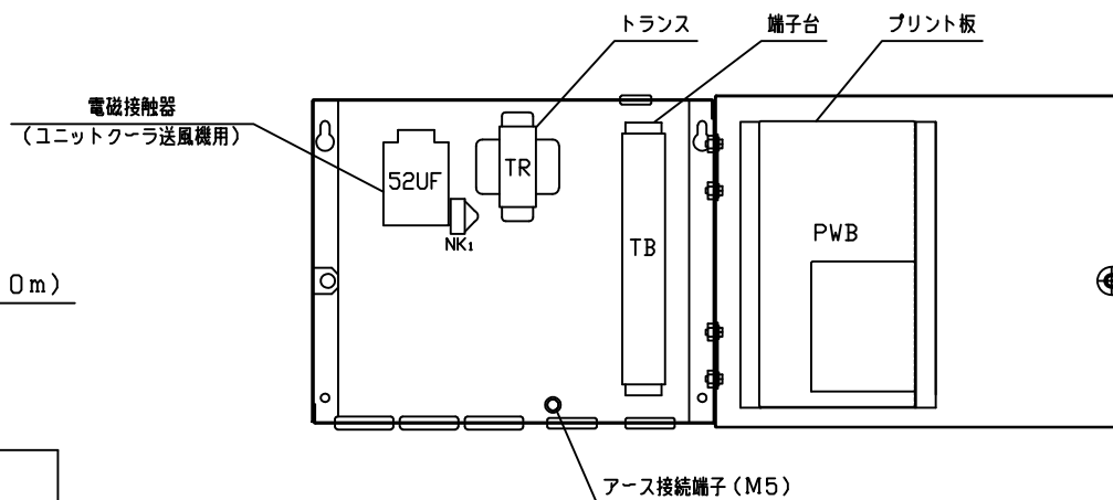
機器配置図
