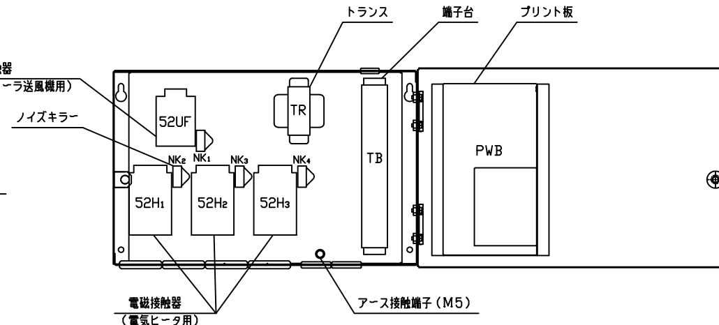
機器配置図
