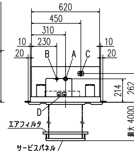
据付スペース
