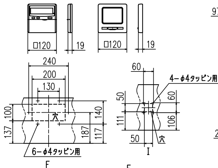
標準リモコン
