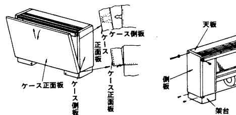
床面固定の場合
