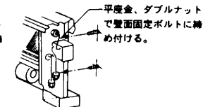
壁面固定の場合
