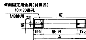
床面固定金具用ボルト位置
