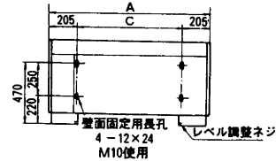
壁面固定用ボルト位置
