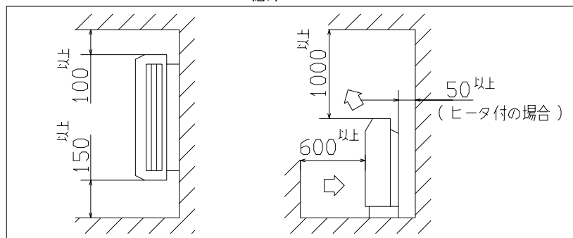
据付スペース
