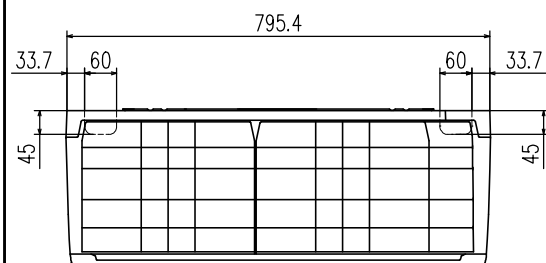
外形図（室内ユニット）
