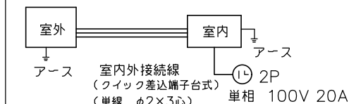
配線接続図
