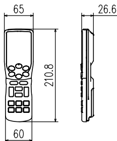
外形図（リモコン）
