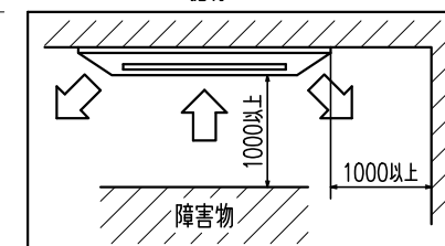
据付スペース
