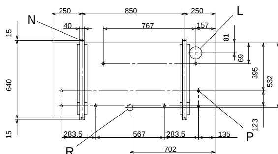
冷媒配管接続口の寸法 (平面図)
