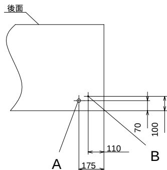
冷媒配管接続口の寸法 (平面図)
