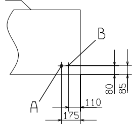
冷媒配管接続口の寸法 (平面図)
