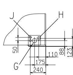
冷媒配管接続口の寸法 (正面図)
