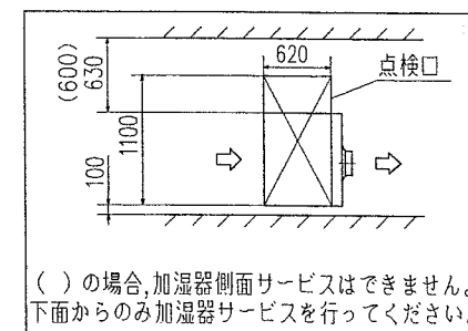
据付スペース
