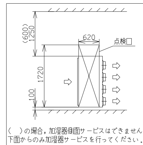
据付スペース
