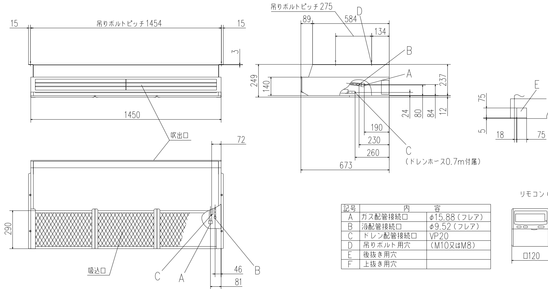
据付スペース
