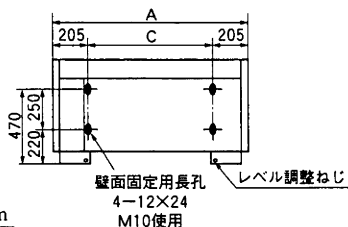
壁面固定用ボルト位置
