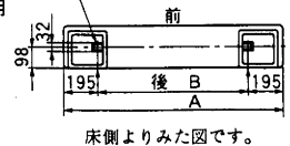
床面固定金具用ボルト位置
