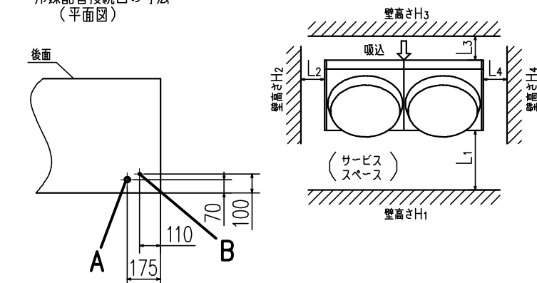
冷媒配管接続口の寸法 (平面図)
