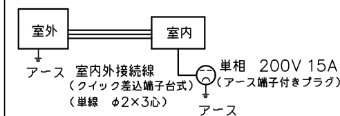
配線接続図
