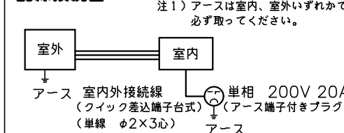
配線接続図
