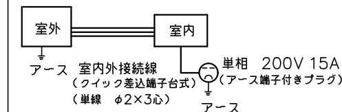
配線接続図
