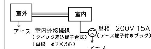
配線接続図
