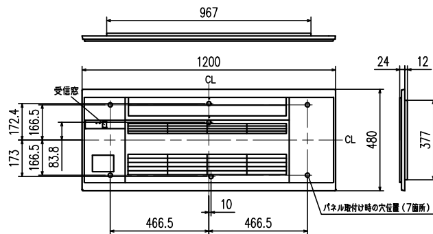
化粧パネル外形図 (TTPN-23W-R,23C-R,23M-R,23T-R)
