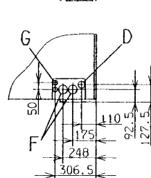
冷暖配管接続口の寸法 (正面図)
