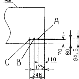
冷暖配管接続口の寸法 (平面図)
