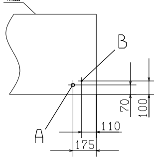
冷媒配管接続口の寸法 (後面)
