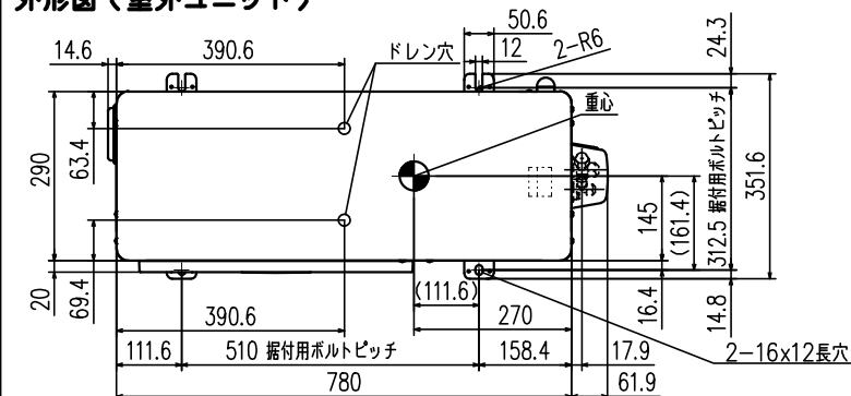
外形図（室外ユニット）
