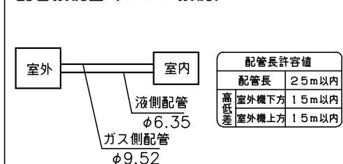
配管接続図（フレア接続）
