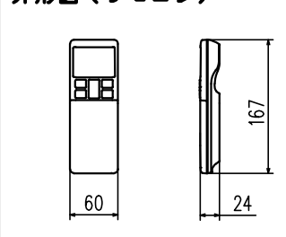
外形図（リモコン）
